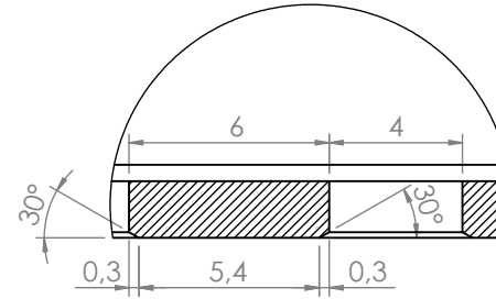
C (4 : 1)
