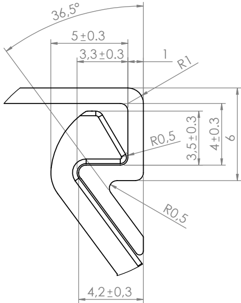
A (4 : 1)
